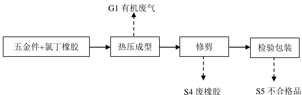
图 5-2 低压柜配件（手柄、隔弧板、导线圈）生产工艺流程图
