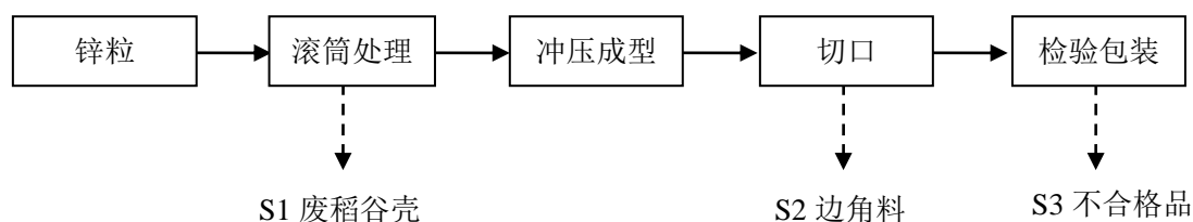
图 5-1 电池配件（锌筒）生产工艺流程图
