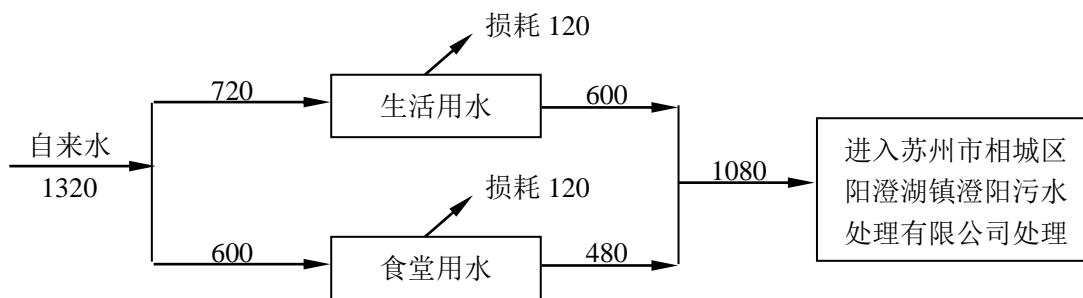
图 5-5 本项目水平衡图 (t/a)
