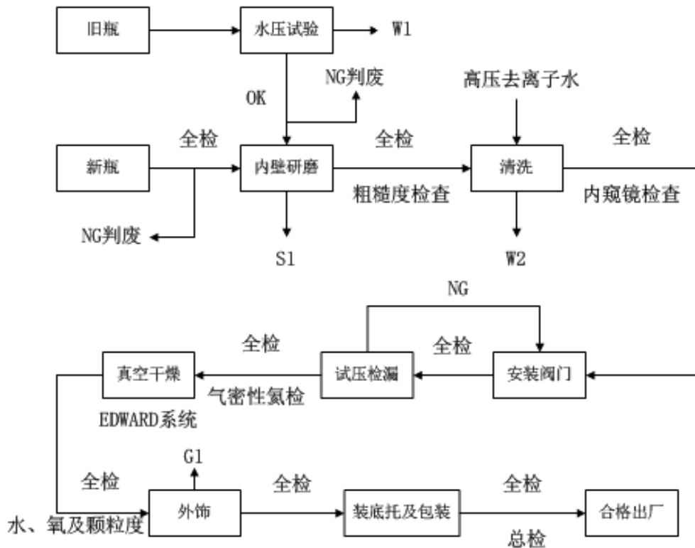
图 1-1（超）高纯气体钢瓶处理工艺流程图
