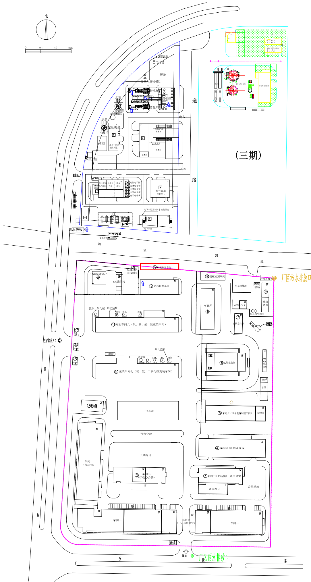
附图五 厂区总平面布置图
