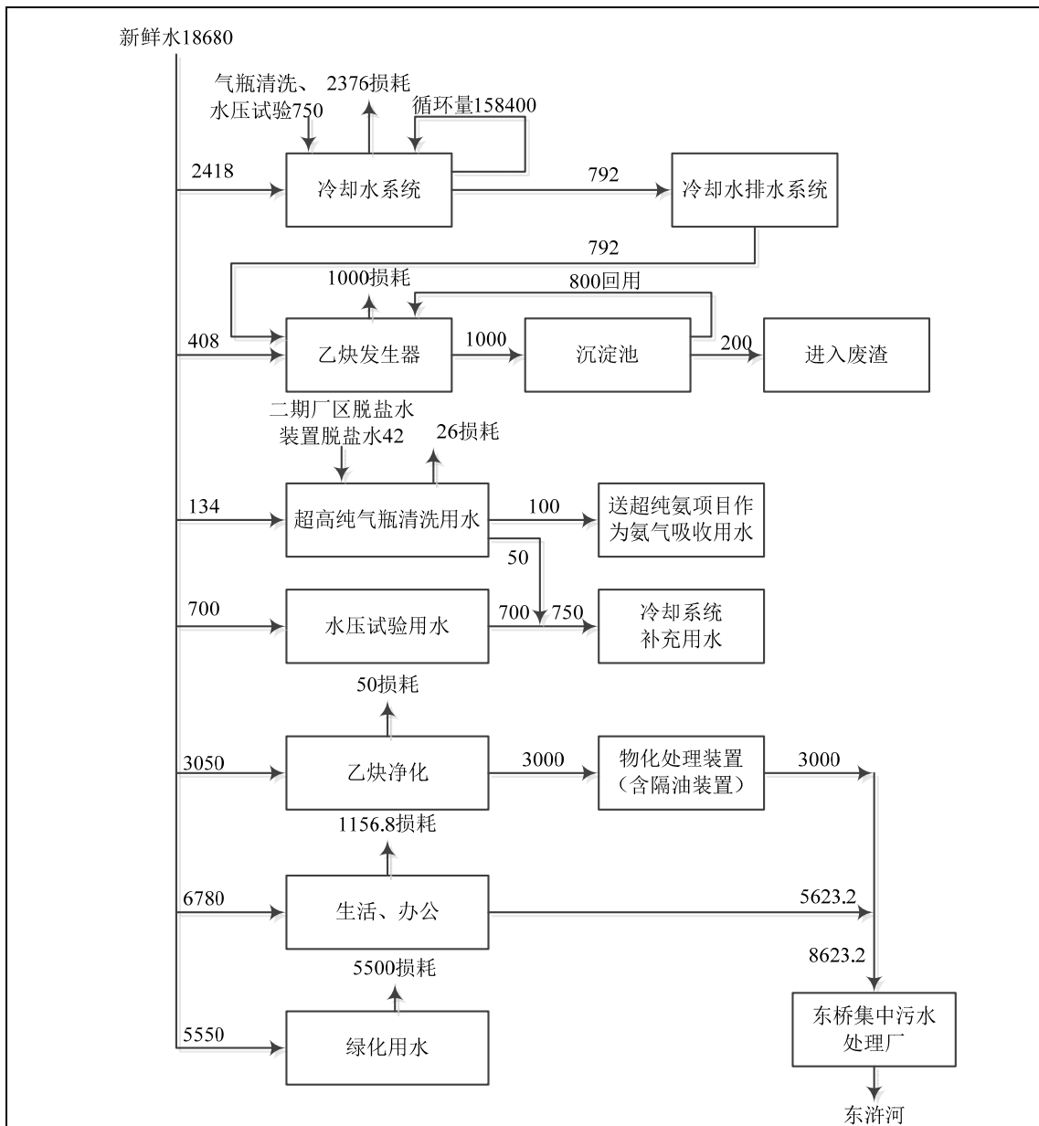
图 5-3 本项目扩建后一期厂区水平衡图 (m 3 /a)
