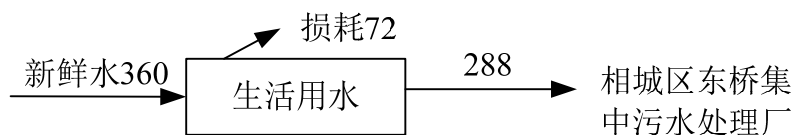
图 5-2 本项目水平衡图 (m 3 /a)
