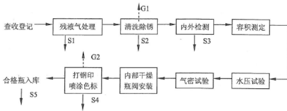
图 1-2 焊接气瓶瓶检工艺流程图
