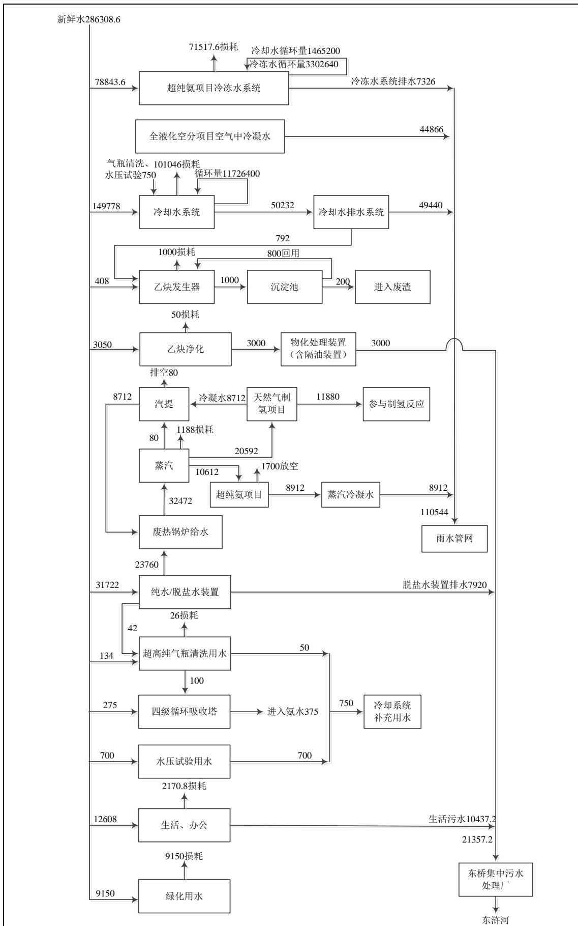
图 5-3 扩建后全厂水平衡图 (m 3 /a)
