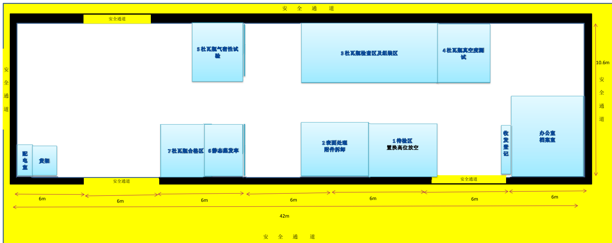
附图六 检测车间平面布置图
