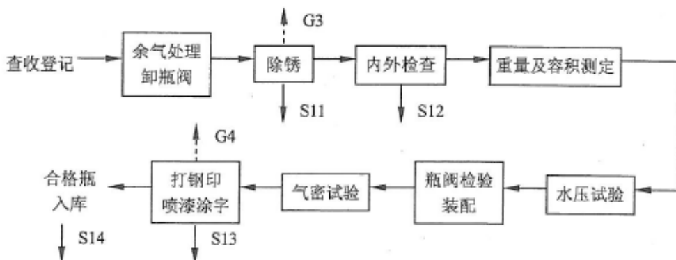
图 1-3 乙炔气瓶瓶检工艺流程图
