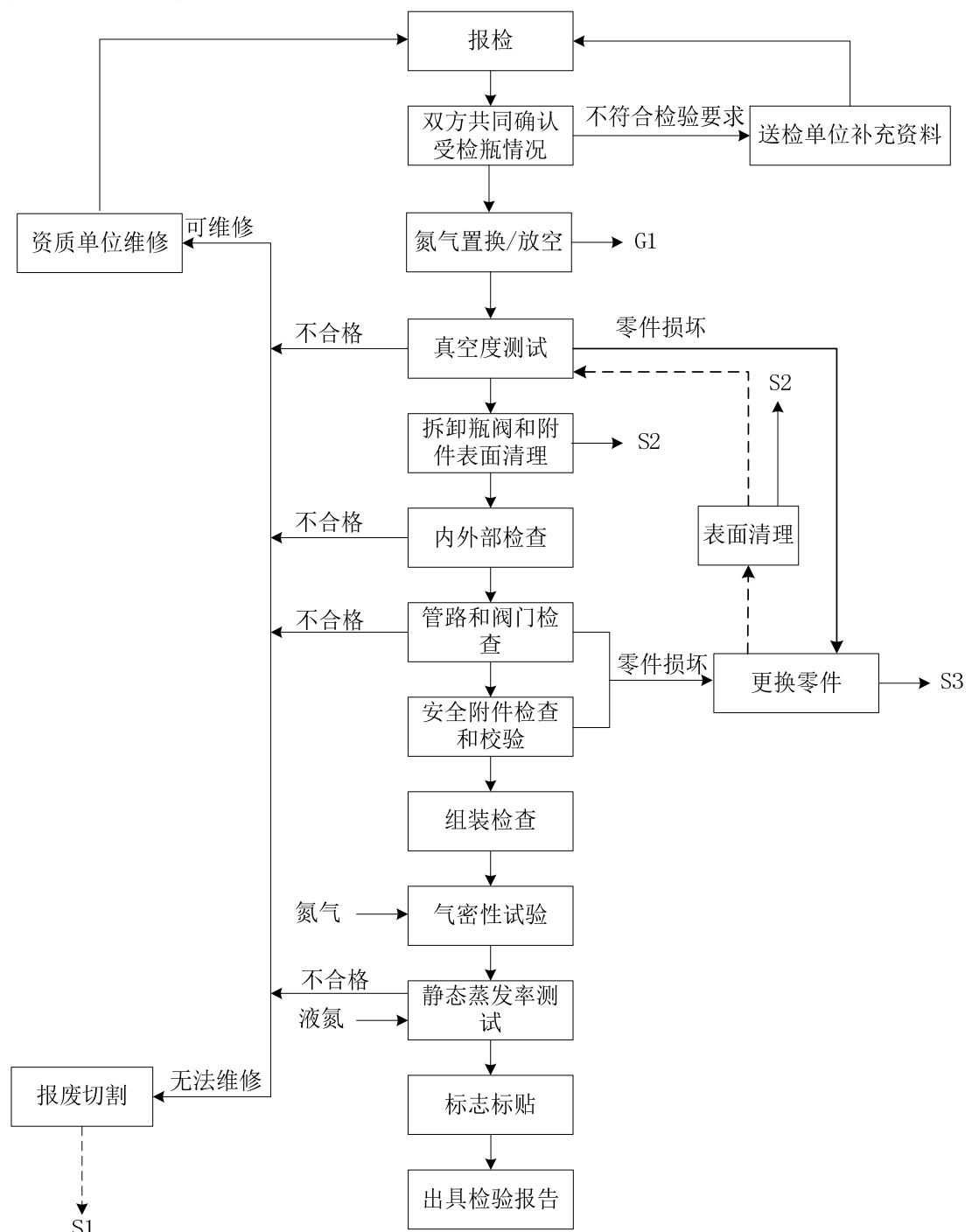
图 5-1 低温绝热气瓶检测生产工艺流程图
