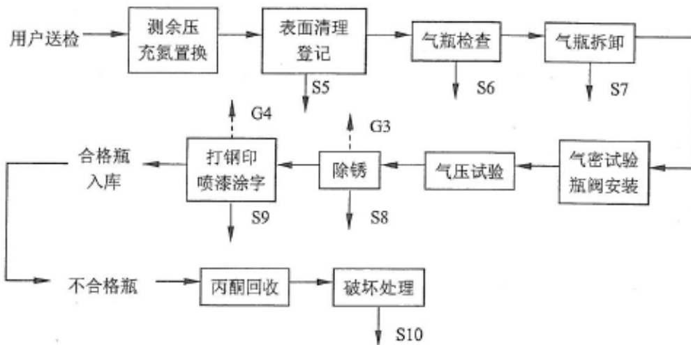
图 1-3 乙炔气瓶瓶检工艺流程图
