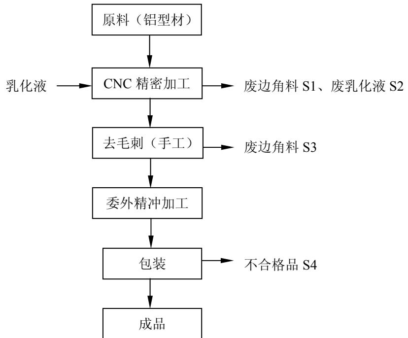
图 1 生产工艺流程图
